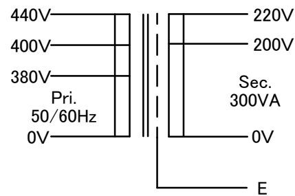
結線図
