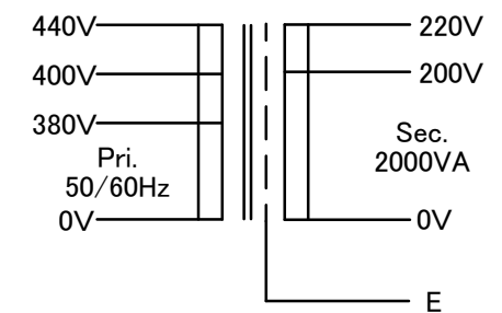
結線図
