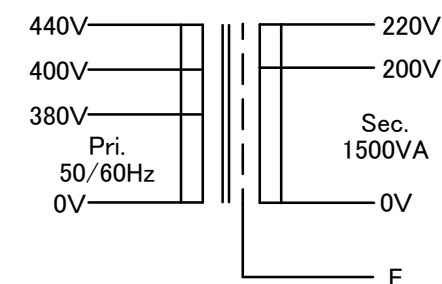
結線図
