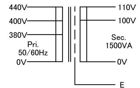
結線図
