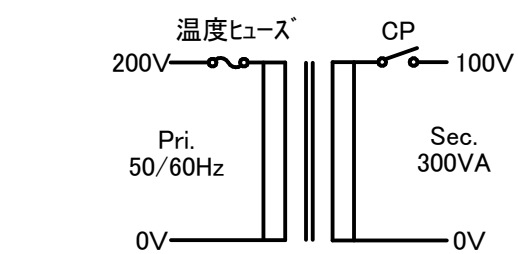
結線図
