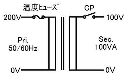
結線図
