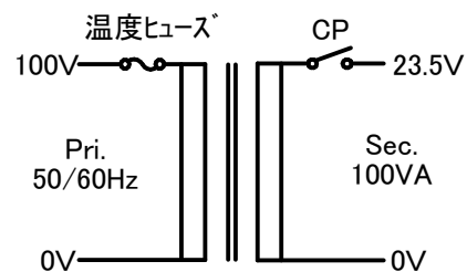
結線図
